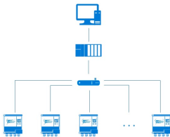
星型拓扑结构
